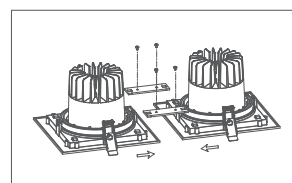
Conexión modular
