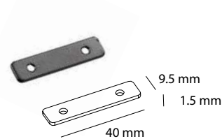
Conector inferior
