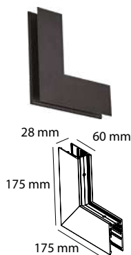
Esquina externa de sobreponer / suspender
