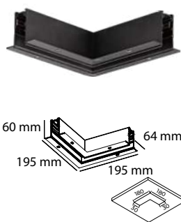
Esquina de empotrar
