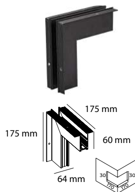
Esquina externa de empotrar
