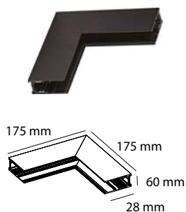
Esquina interna de sobreponer / suspender
