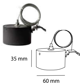
Accesorio de suspender
