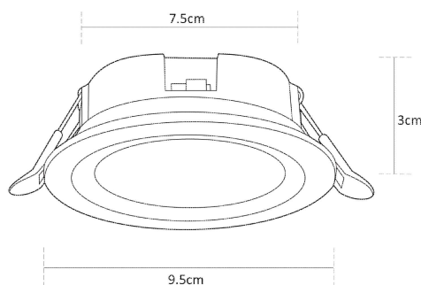
Diagrama de dimensiones
