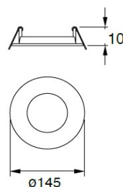
Dimensiones en milímetros
