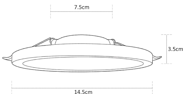
Diagrama de dimensiones
