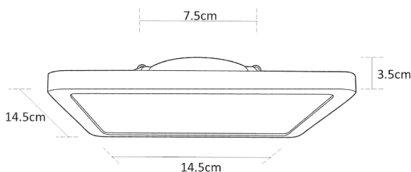
Diagrama de dimensiones
