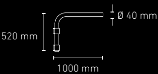
BRAZO METÁLICO LARGO Ø 40 mm
