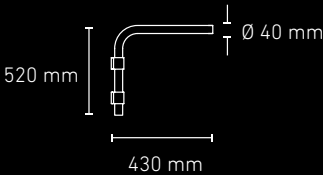
BRAZO METÁLICO MEDIANO Ø 40 mm
