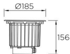
Dimensiones en milímetros
