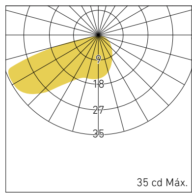
5.1 EFICIENCIA DEL SISTEMA: 34 lm/W @ 2700 K 41 lm/W @ 4000 K
