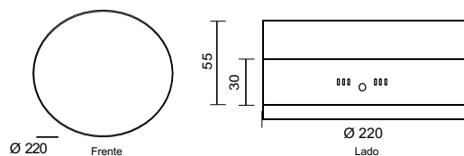
DIAGRAMA DE DIMENSIONES:
