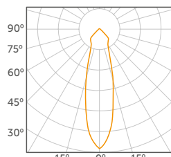
REFLECTOR MEDIO 26°
