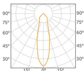
REFLECTOR MEDIO 26°
