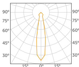
REFLECTOR CONCENTRADO 19°
